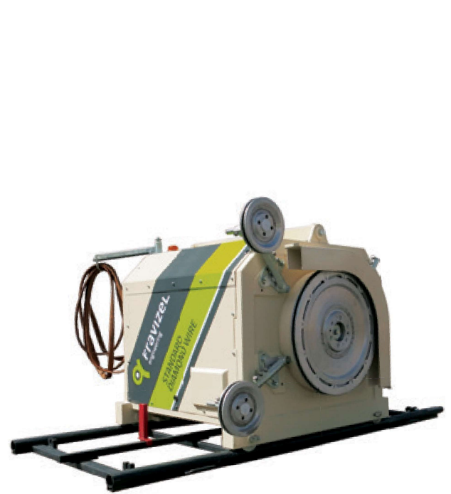
49 MÁQUINA DE FIO STANDARD 40/50/60 CV (MFS) STANDARD DIAMOND WIRE MACHINE 40/50/60 HP MAQUINA DE CORTE POR HILO DIAMANTADO ESTÁNDAR 40/50/60 HP SCIE FIL AU DIAMANT STANDARD 40/50/60 HP
